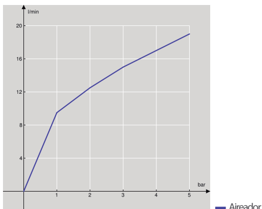
DIAGRAMA DE FLUJO: AGUA MEZCLADA
