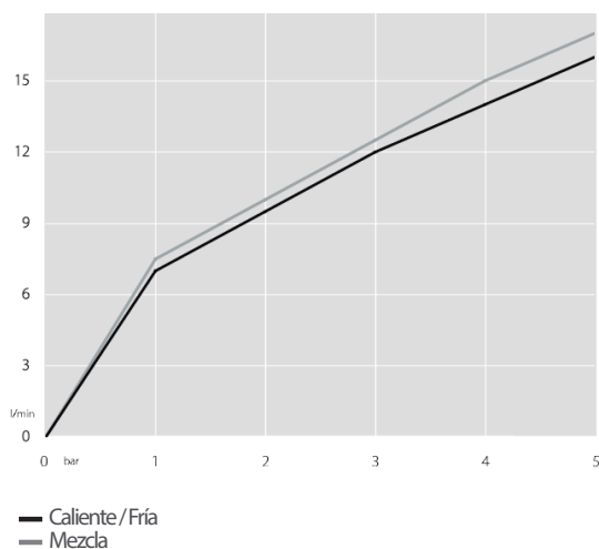
DIAGRAMA DE FLUJO: AGUA CALIENTE/FRIA
